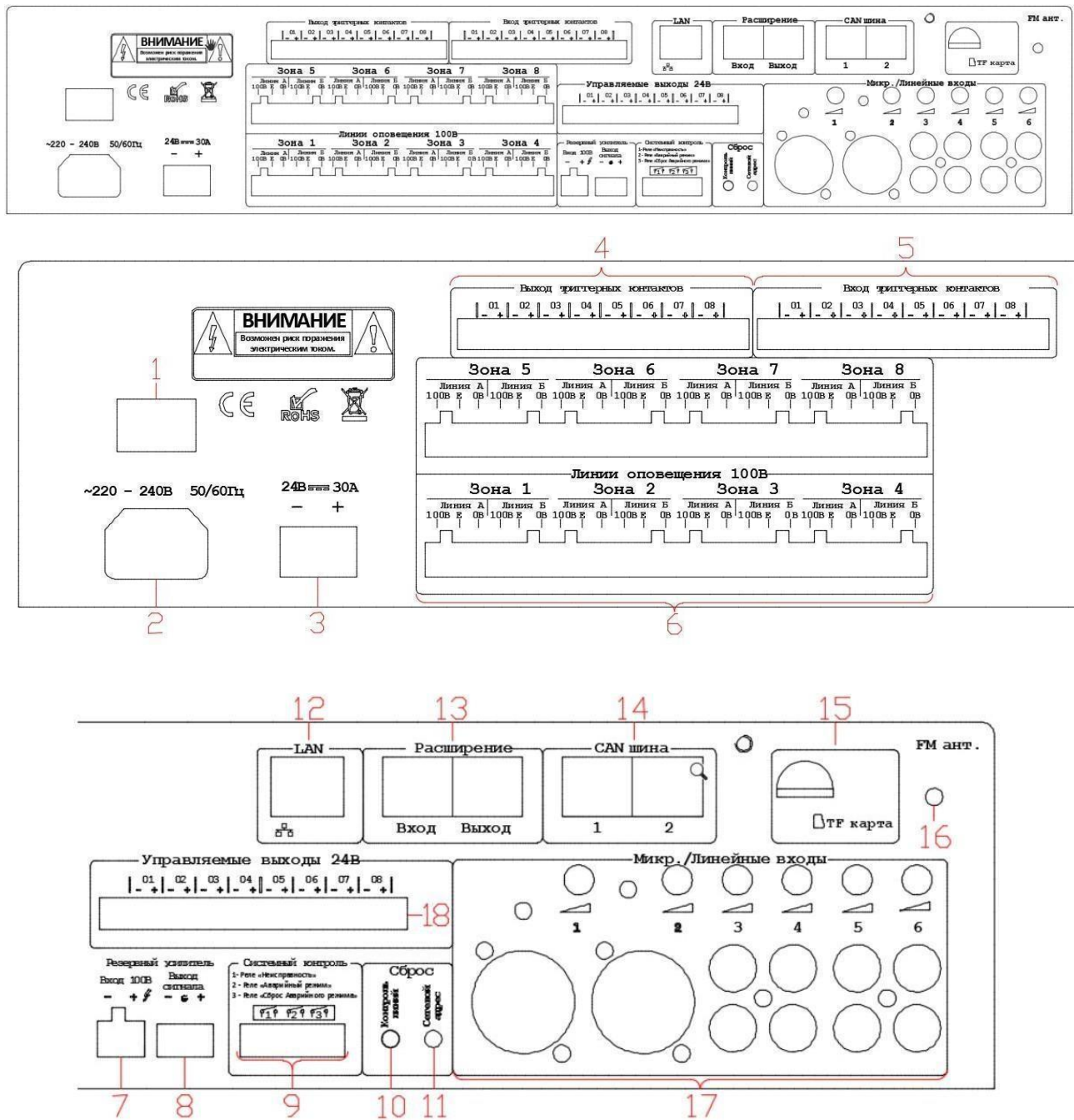
Рис. 2.1.3. Контроллер системы LPA-DUO-M (задняя панель)
